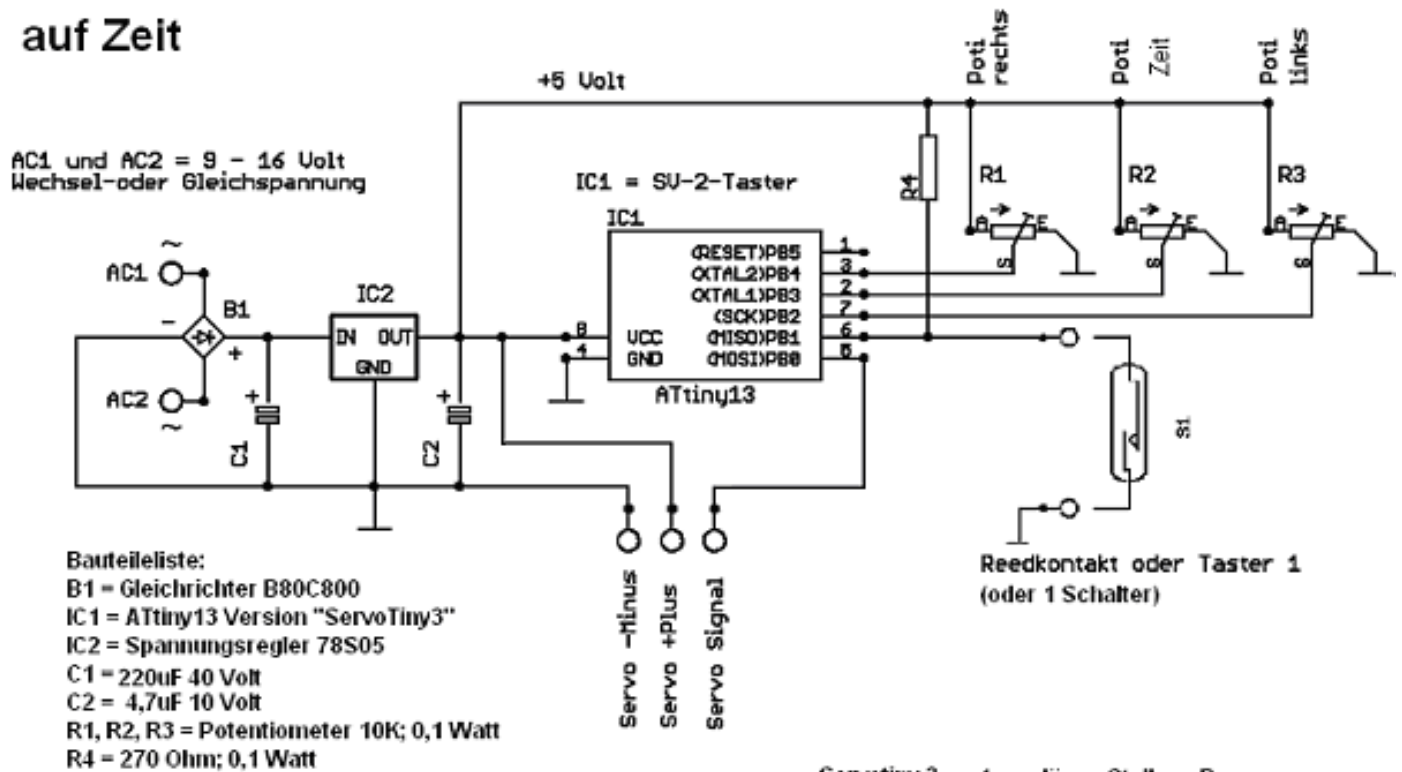
Servotiny 3 1. auslösen Stellung B nach Zeit Stellung A
